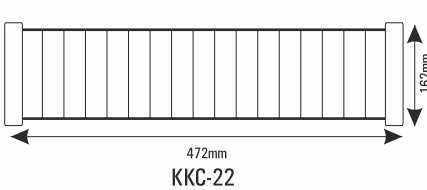
KKC-22
